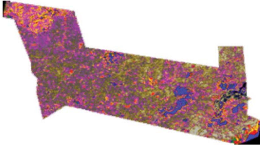
الشكل 6D. خارطة الـ Prod. لشهر مايو 2015.
