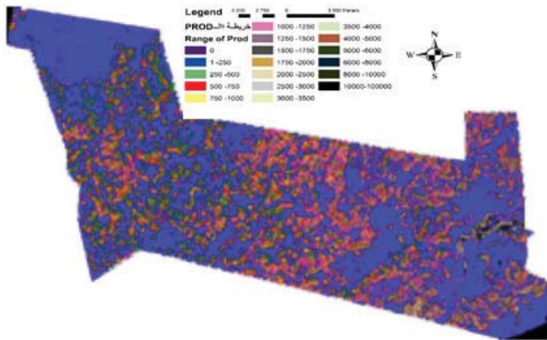
الشكل 8D. خارطة الـ Prod. لشهر مايو 2015.
