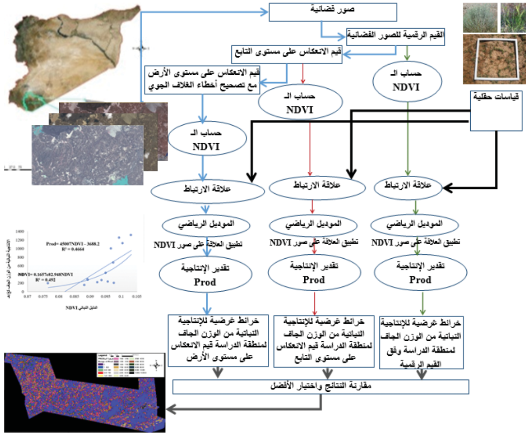
الشكل 1. مخطط يوضح خطوات تنفيذ البحث.
