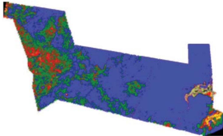
الشكل 6E. خارطة الـ Prod. لشهر يونيو 2015.
