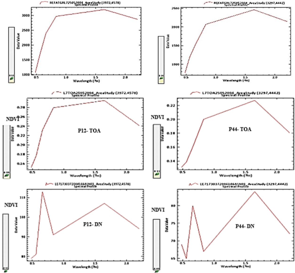
الشكل 2. الاستجابة الطيفية لبيكسل من موقعين حقليين مع قيم الدليل النباتي NDVI.
