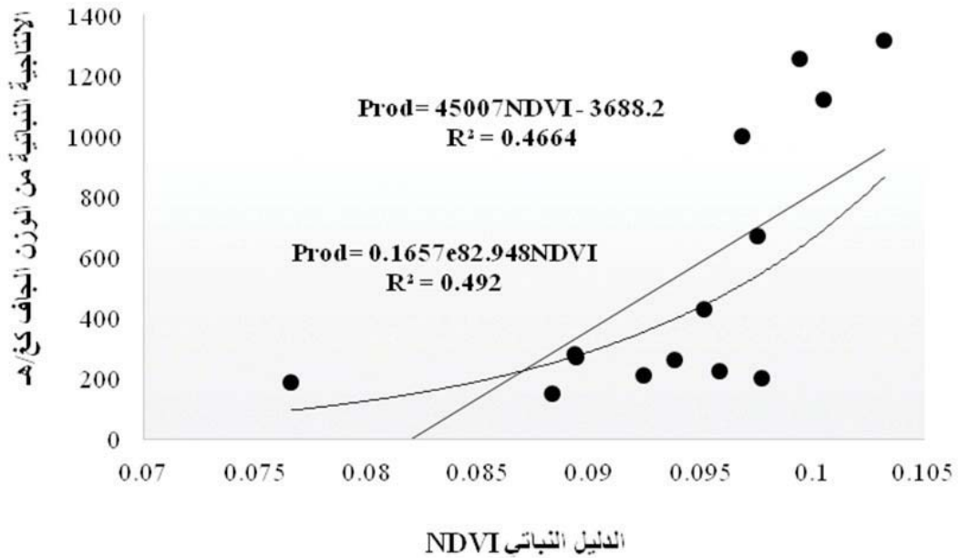
الشكل 5. العلاقة بين Prod والـ NDVI وفق قيم الانعكاس على مستوى التابع.
