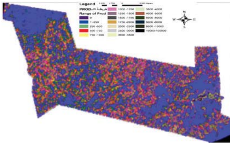
الشكل 8C. خارطة الـ Prod. لشهر أبريل 2015.
