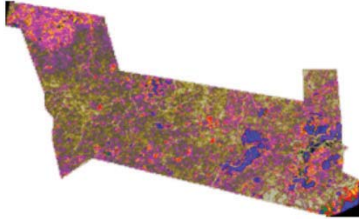
الشكل 6C. خارطة الـ Prod. لشهر إبريل 2015.
