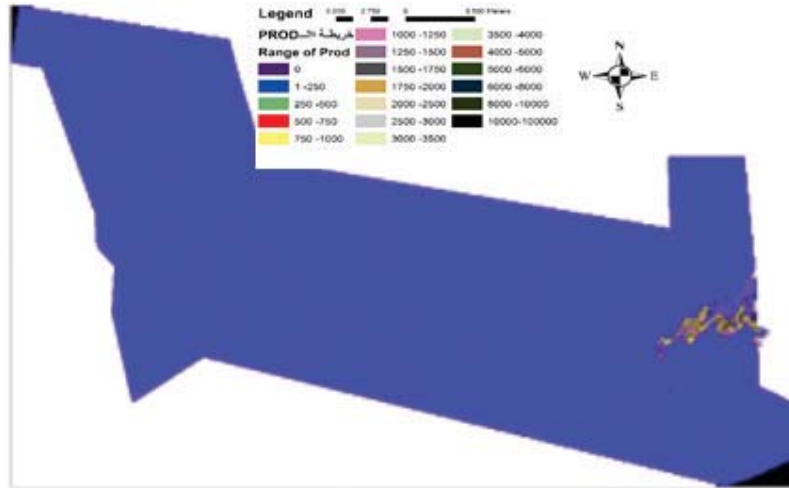
الشكل 8E. خارطة الـ Prod. لشهر يونيو 2015.
