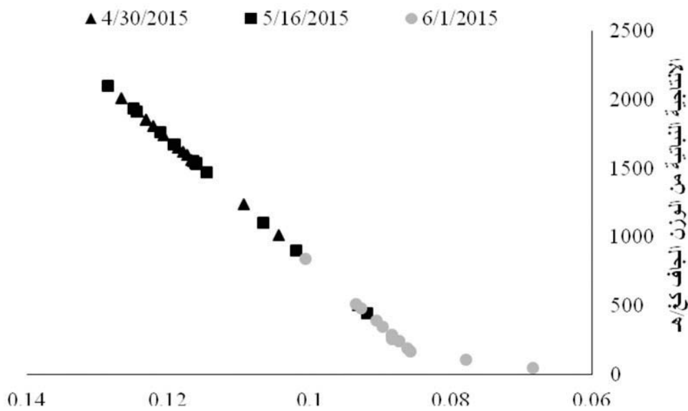
الشكل 6B. تقدير الـProd. لأشهر إبريل ومايو ويونيو 2015.
