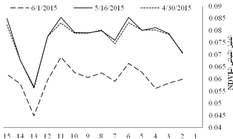
الشكل 4A. تغير قيم NDVI_{MEAN} لأشهر إبريل ومايو ويونيو 2015.
