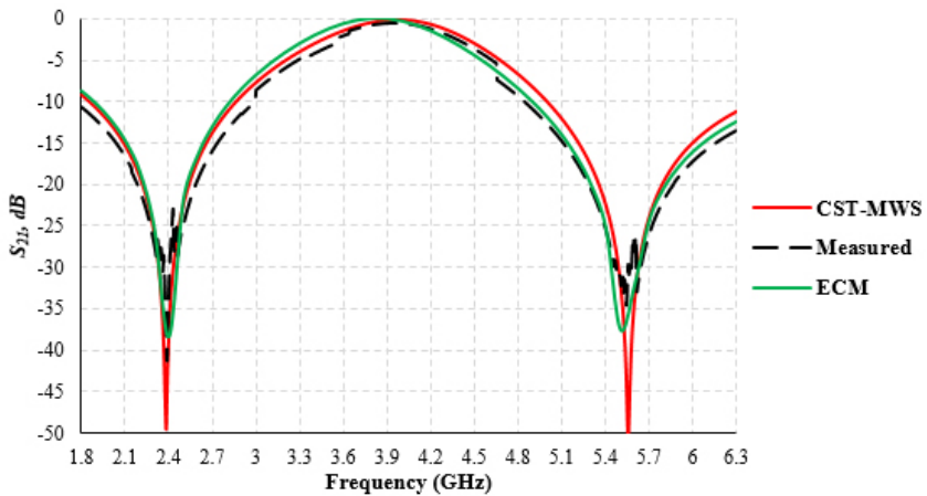
(b) TM-wave
