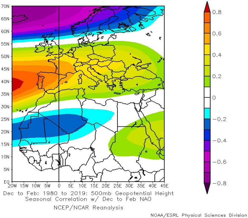
الشكل (8): النمط المكاني لقيم الارتباط بين هطول أمطار (DJF) 500GPCP) وقيم NAO للفترة 1980-2019.
