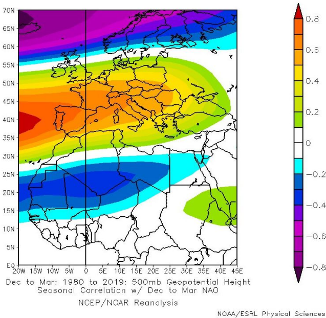
الشكل (11): النمط المكاني لقيم الارتباط بين هطول أمطار (DJFM) 500 GPCP) وقيم NAO للفترة 1980 - 2019.
