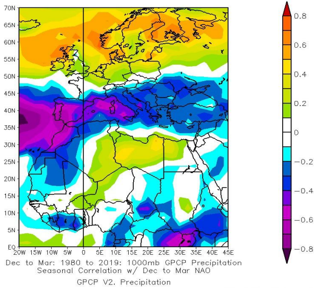
الشكل (10): النمط المكاني لقيم الارتباط بين هطول أمطار (DJFM) 1000 GPCP) وقيم NAO للفترة 1980 - 2019.
