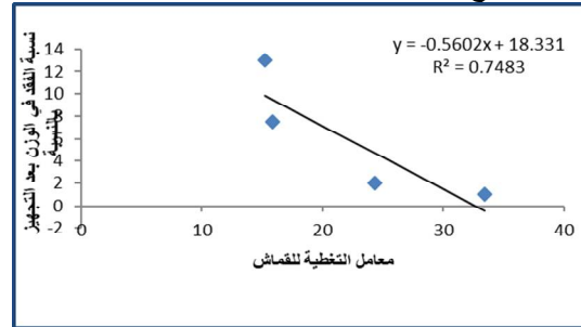
شكل (3) يوضح معادلة خط الانحدار ومعامل الارتباط لمتغيرات البحث مع نتائج اختبار مقاومة الاحتكاك قبل التجهيز
