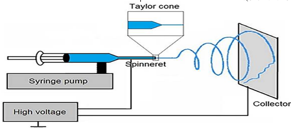
شكل 1: رسم تخطيطي لنظام الغزل الكهربائي (Haider, S: 2016)
