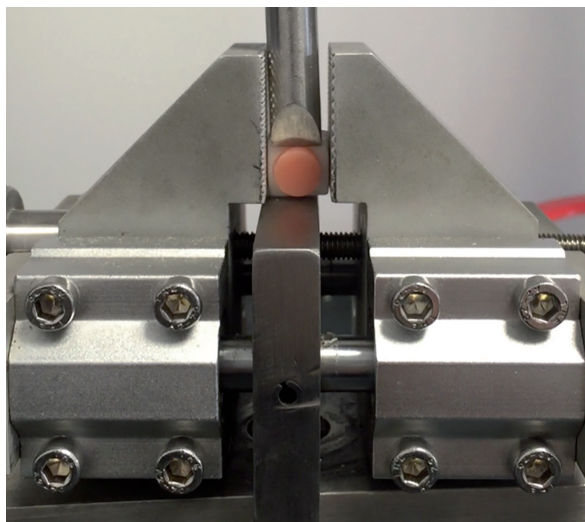
Fig. 3: application des forces de cisaillement à l'interface substrat/résine composite.
