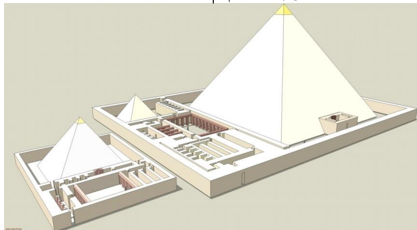
(شكل 5) مسقط افقي ثلاثي الأبعاد للمعبد الجنائزي لمقبرة الملك أوسر كاف
